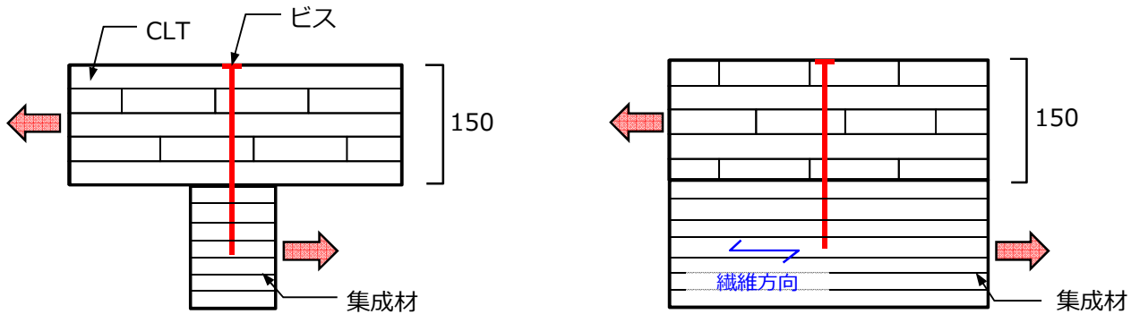
[C - 1]CLT-集成材接合(繊維直交方向せん断)
